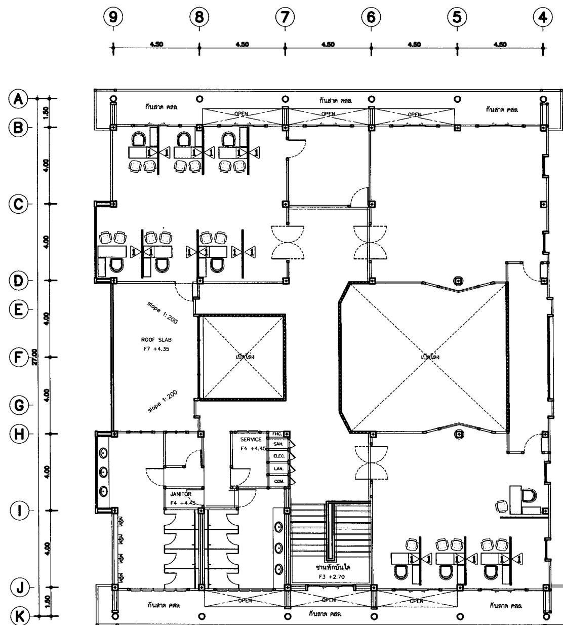
แปลนการจัดพื้นที่ภายในห้องชั้นที่ 2 มาตรฐาน 1 : 200
