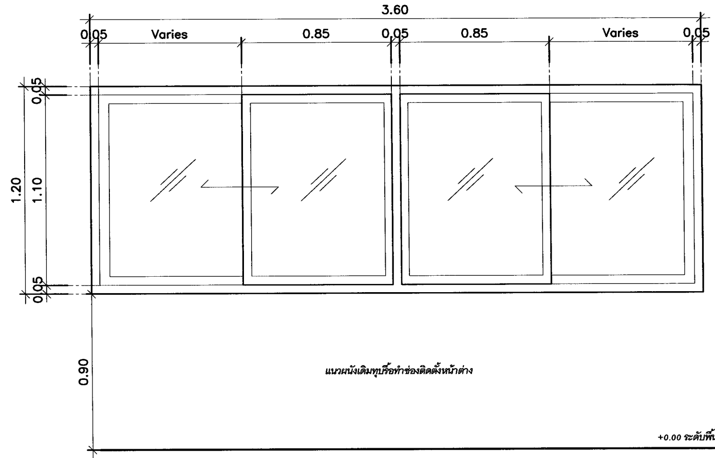
แบบขยายหน้าต่าง 1
