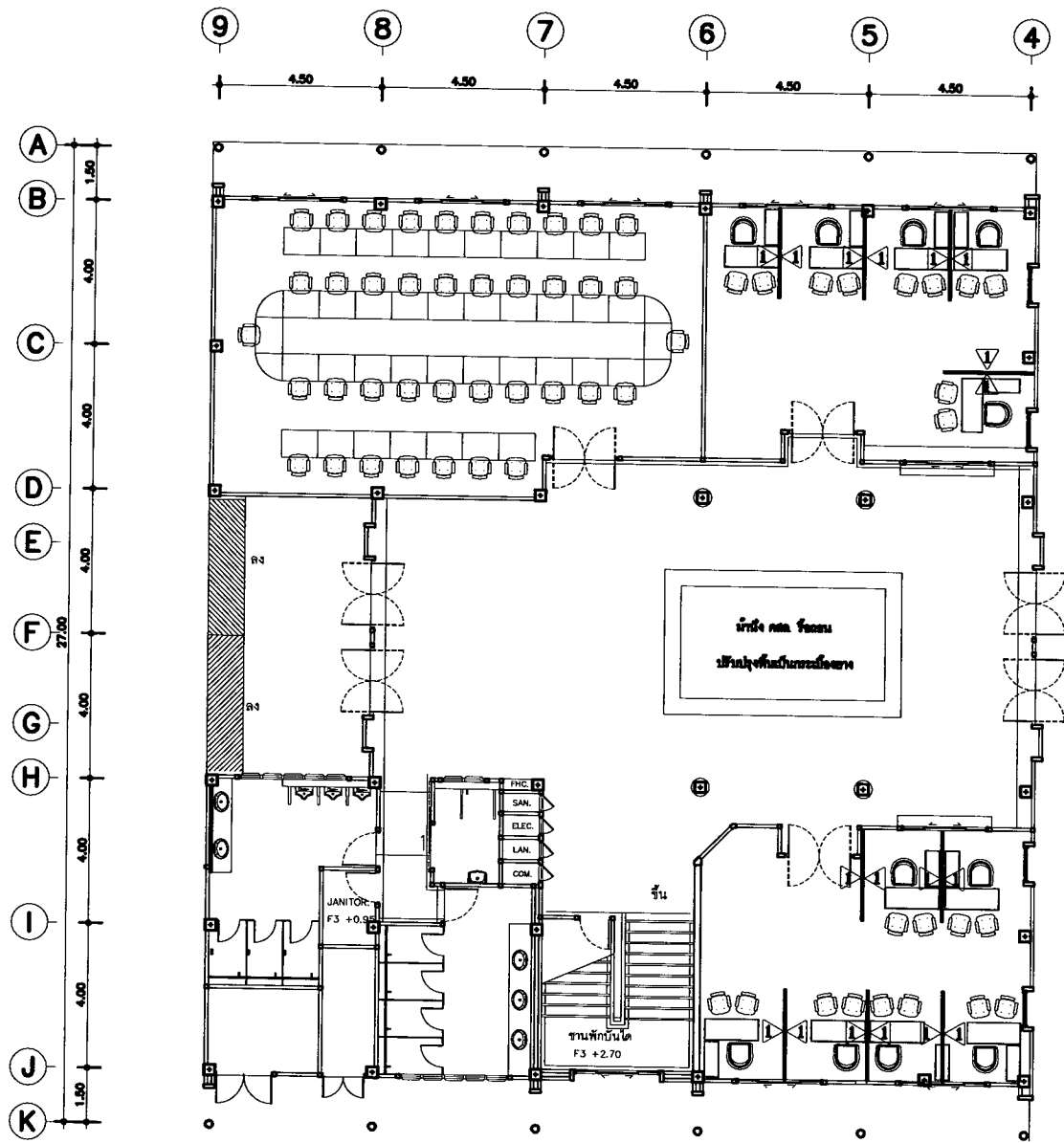
แปลนการจัดพื้นที่ภายในห้องชั้นที่ 1 มาตรฐาน 1 : 200
